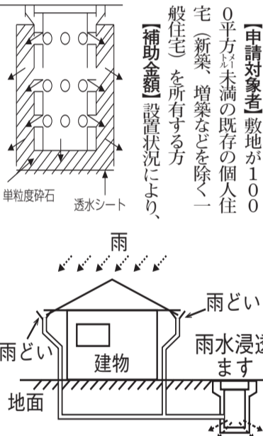
雨水浸透ますの構造と設置の仕組み
