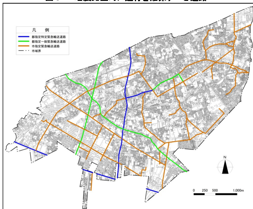
図 3-1 地震発生時に通行を確保すべき道路
