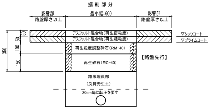
標準構造図 35型-B
