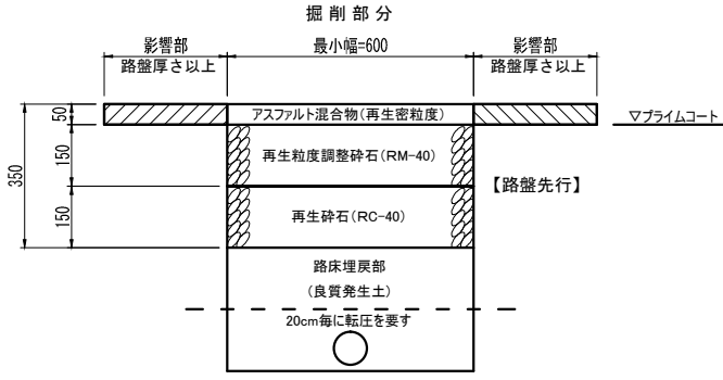
標準構造図 35型-A
