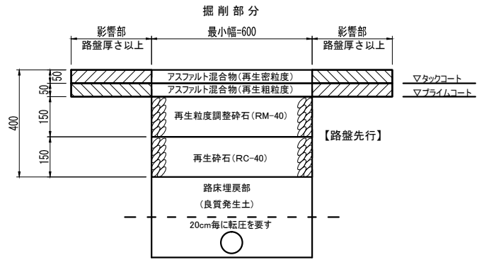
標準構造図 40型
