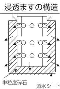
雨水浸透のしくみ
