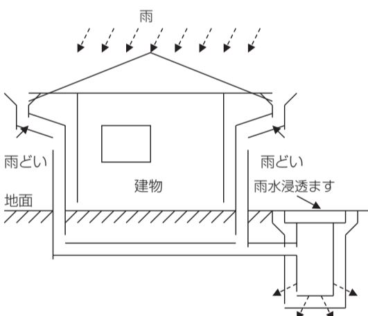
雨水浸透のしくみ
